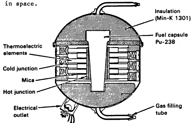
Fig. 1 SNAP-3B RTG
